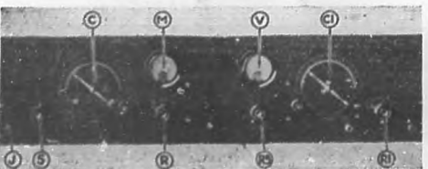
Vista del frente del receptor de 10 válvulas. C. y C-1 son los cuadrantes de sintonización. La selectividad del circuito de antena puede aumentarse o disminuirse con el empleo del conmutador S. En el enchufe J puede conectarse una antena de cuadro.
