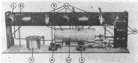
El receptor de diez válvulas, mostrando los transformadores radiofrecuenciales L-1, el condensador de sintonización de la antena C, y los condensadores de sintonización radiofrecuente C-1, que forman una sola unidad. Los transformadores radiofrecuenciales son del tipo de enchufe, de manera que el receptor puede cubrir una banda de ondas desde 35 hasta 3600 metros.
